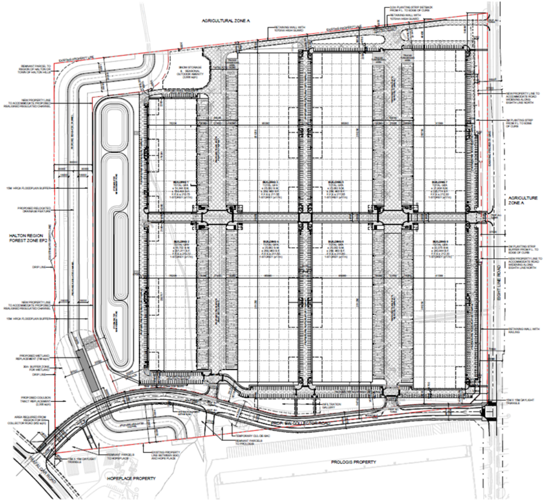
1 SITE PLAN A103 1:1500
